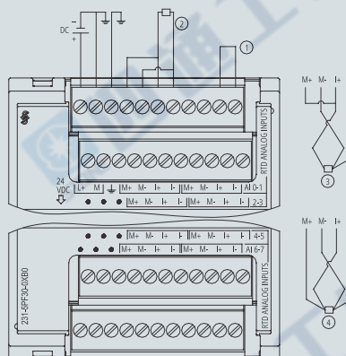
SM 1231 8 x 16 位热电阻模拟量输入
